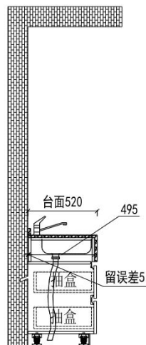
2F主卫侧视图
