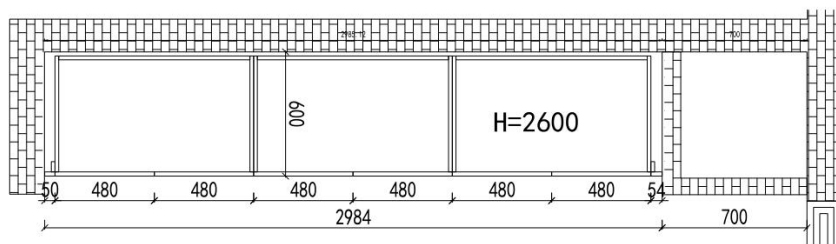
2F主卧衣帽间俯视图 (A面)
