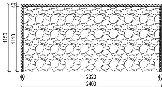
1F厨房岛台外视图（餐厅面）
