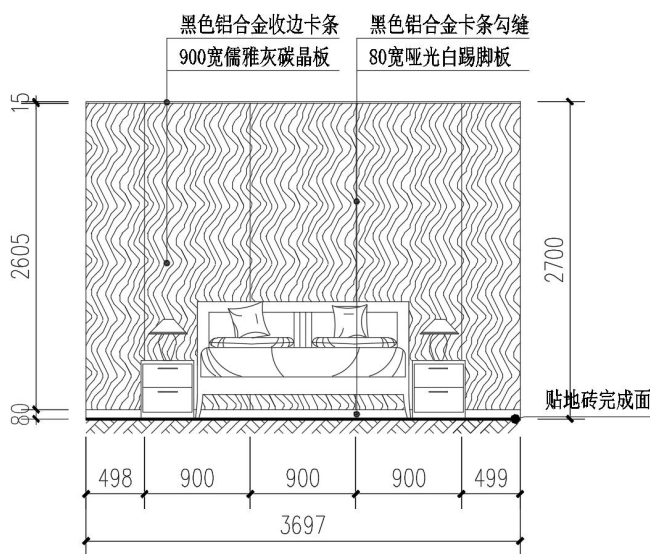
一层卧室D墙立面图 1:50
