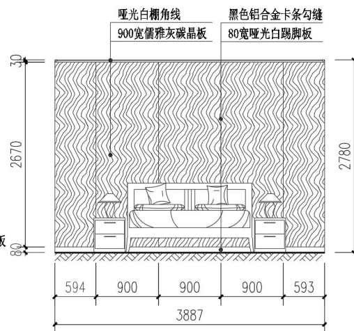
二层主卧室C墙立面图 1:50
