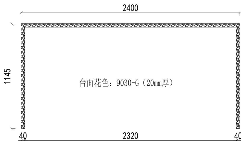
1F西厨岛台立面图
