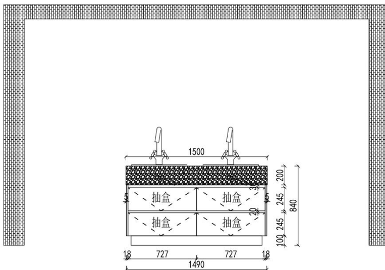
2F主卫外视图
