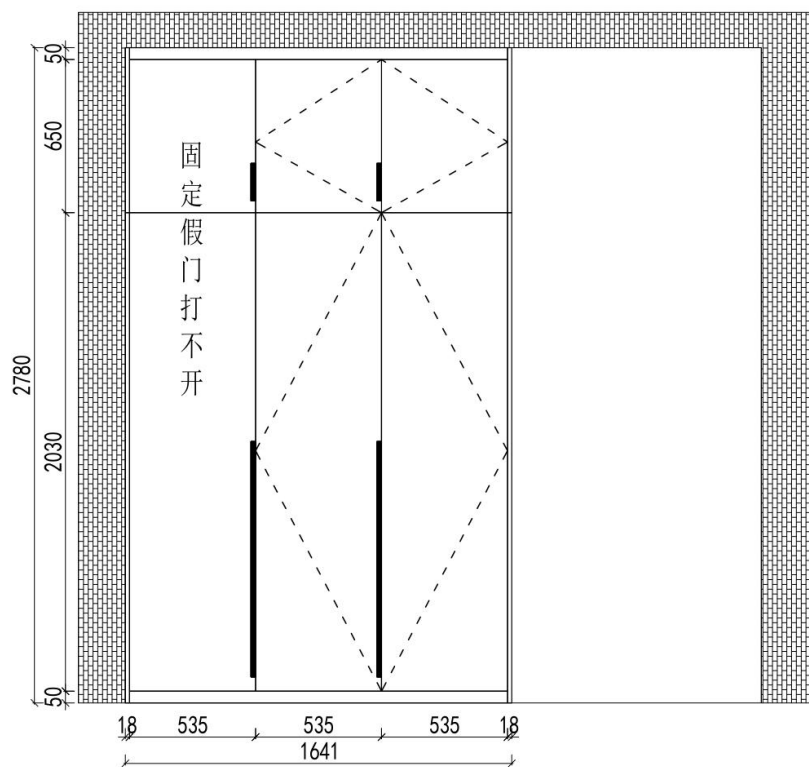
2F儿童房衣柜外视图
