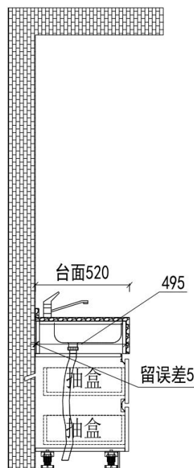
2F卧室3卫生间侧视图
