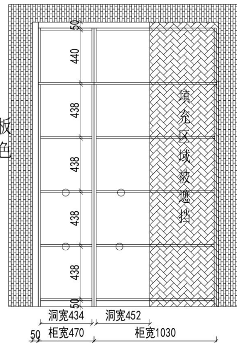
1F储藏间外视图B
