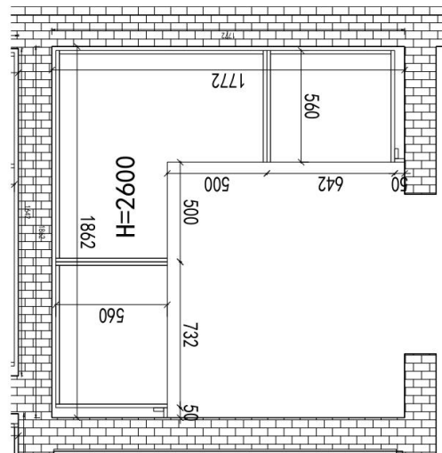
1F卧室1衣帽间俯视图
