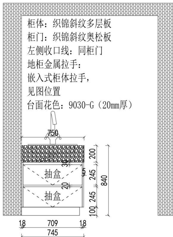
1F卧室1卫生间外视图
