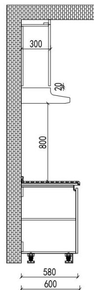
1F厨房侧视图
