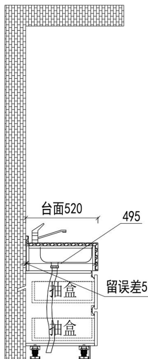
1F卧室1卫生间侧视图
