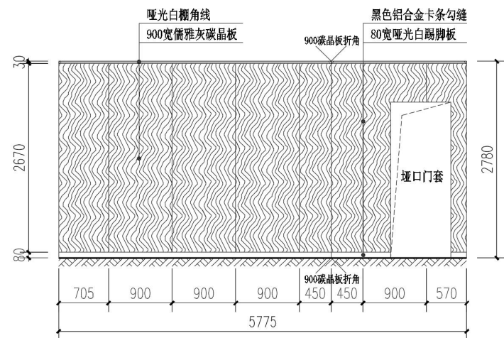
二层起居室B-A立面图 1:50
