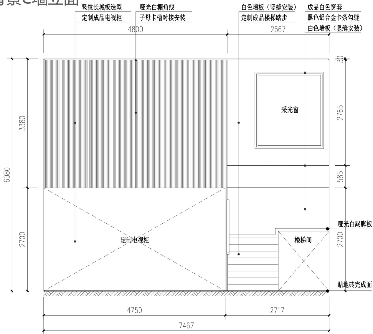
一层电视背景C墙立面图 1:50
