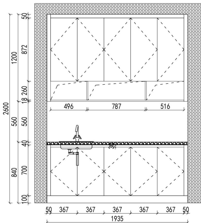
1F洗衣房外视图
