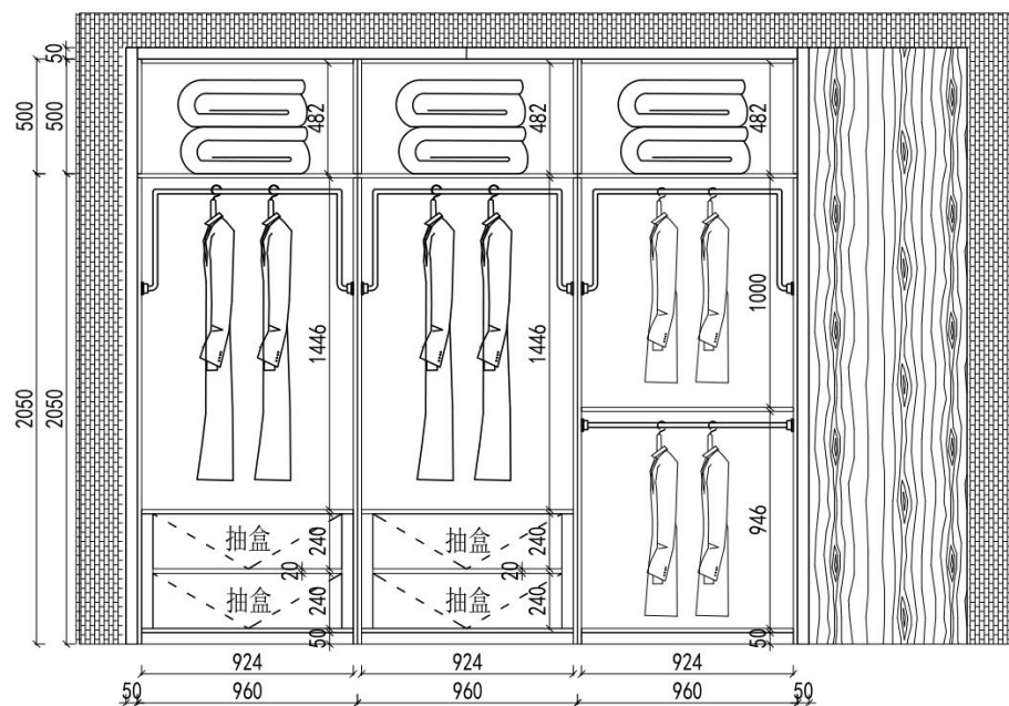
2F主卧衣帽间结构图 (A面)
