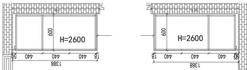
2F主卧衣帽间俯视图 (B面)
