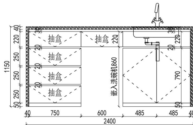
1F厨房岛台外视图（厨房面）
