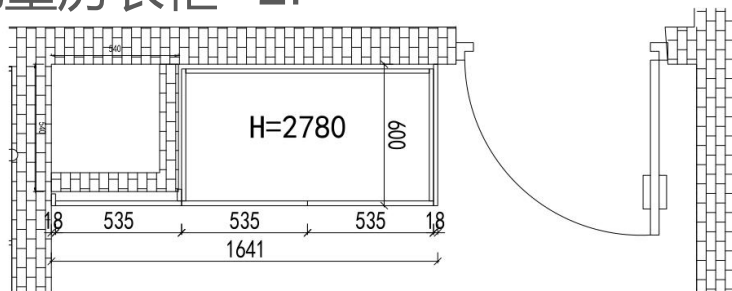
2F儿童房衣柜俯视图
