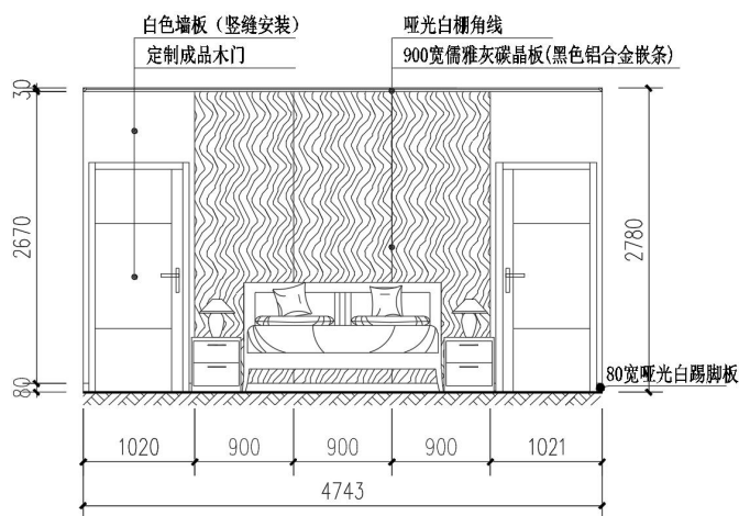
二层卧室3-B墙立面图 1:50
