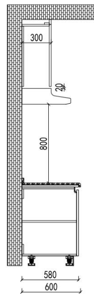
1F厨房侧视图
