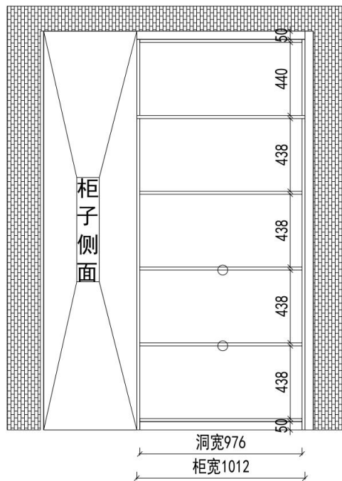
1F储藏间外视图A
