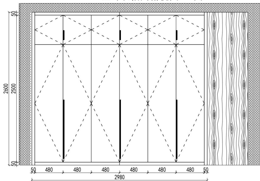
2F主卧衣帽间外视图 (A面)
