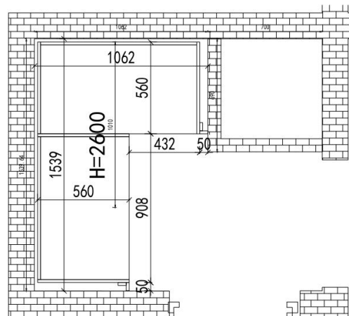
2F卧室2衣帽间俯视图
