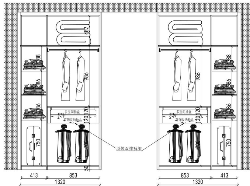
2F主卧衣帽间结构图 (B面)
