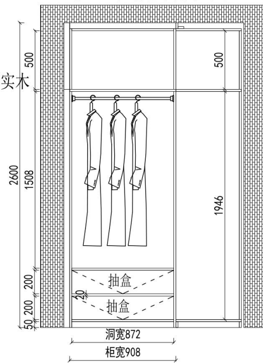
2F卧室2衣帽间外视图B
