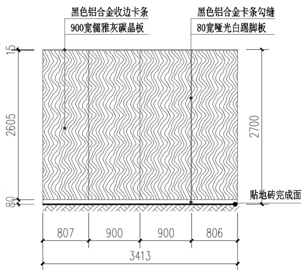
一层书房B墙立面图 1:50
