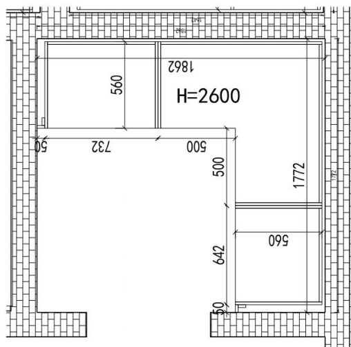
1F卧室1衣帽间俯视图
