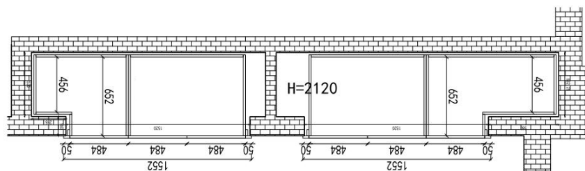
1F客厅衣柜俯视图
