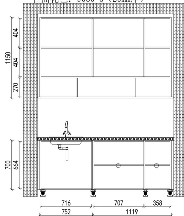
1F洗衣房结构图
