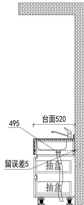
2F卧室2卫生间侧视图
