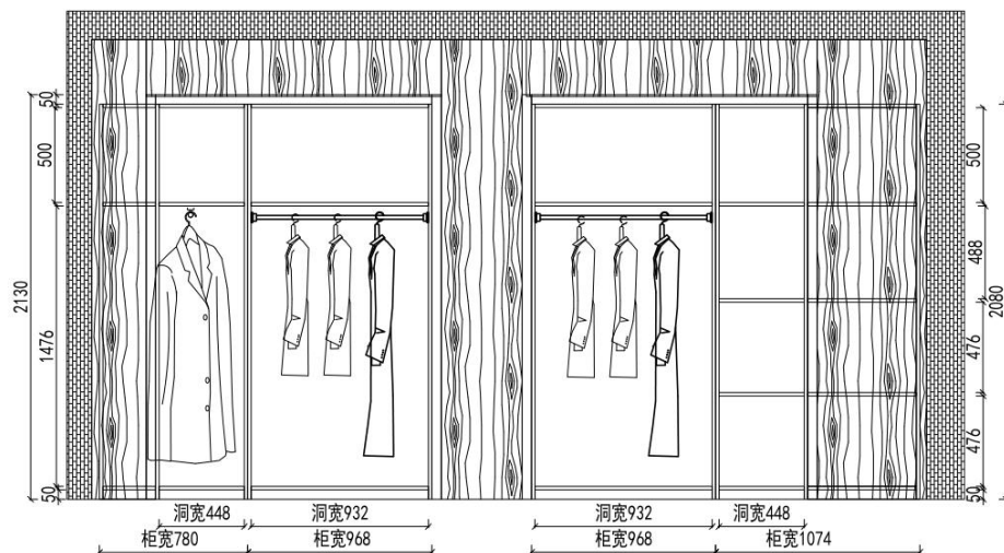
1F客厅衣柜结构图
