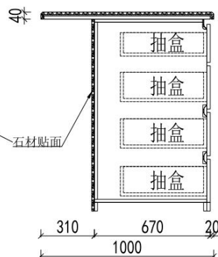
1F厨房岛台侧视图
