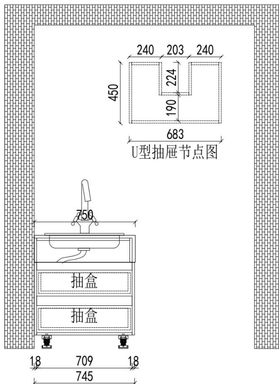
2F卧室2卫生间结构图
