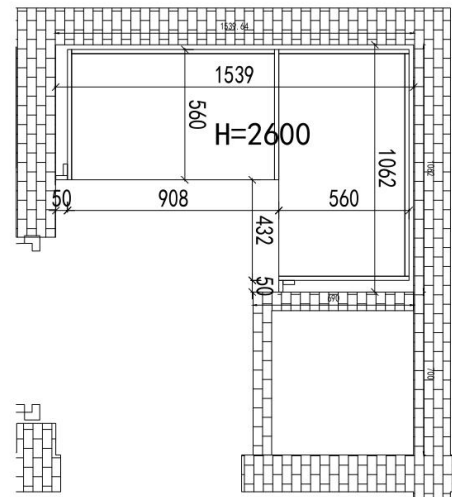
2F卧室2衣帽间俯视图
