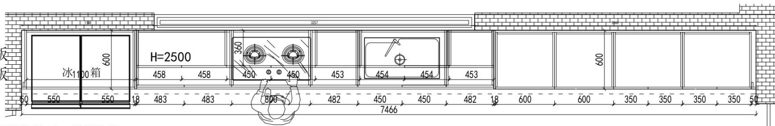
1F厨房俯视图
