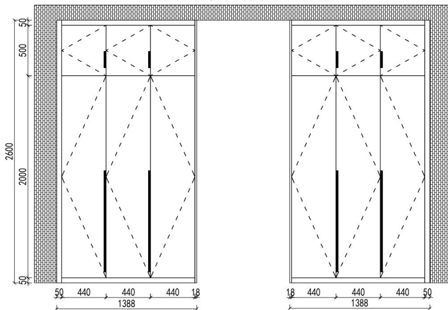
2F主卧衣帽间外视图 (B面)
