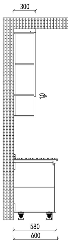
1F洗衣房侧视图
