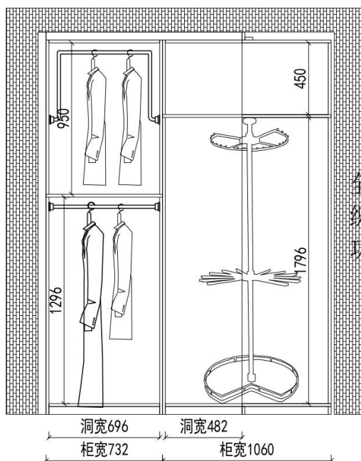
1F卧室1衣帽间外视图A
