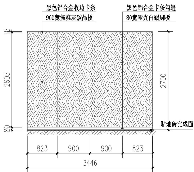
一层小客厅B墙立面图 1:50
