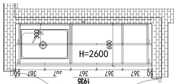
1F洗衣房俯视图
