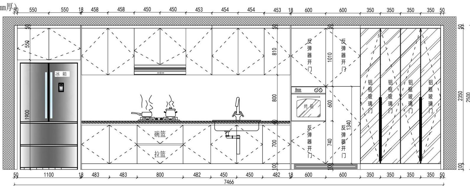
1F厨房外视图
