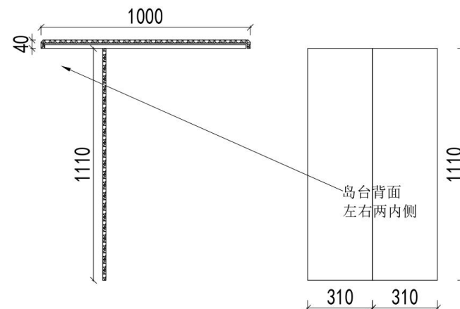
1F西厨岛台侧视图
