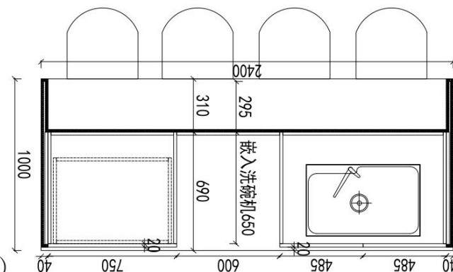
1F厨房岛台俯视图
