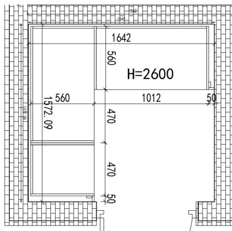
1F储藏间俯视图
