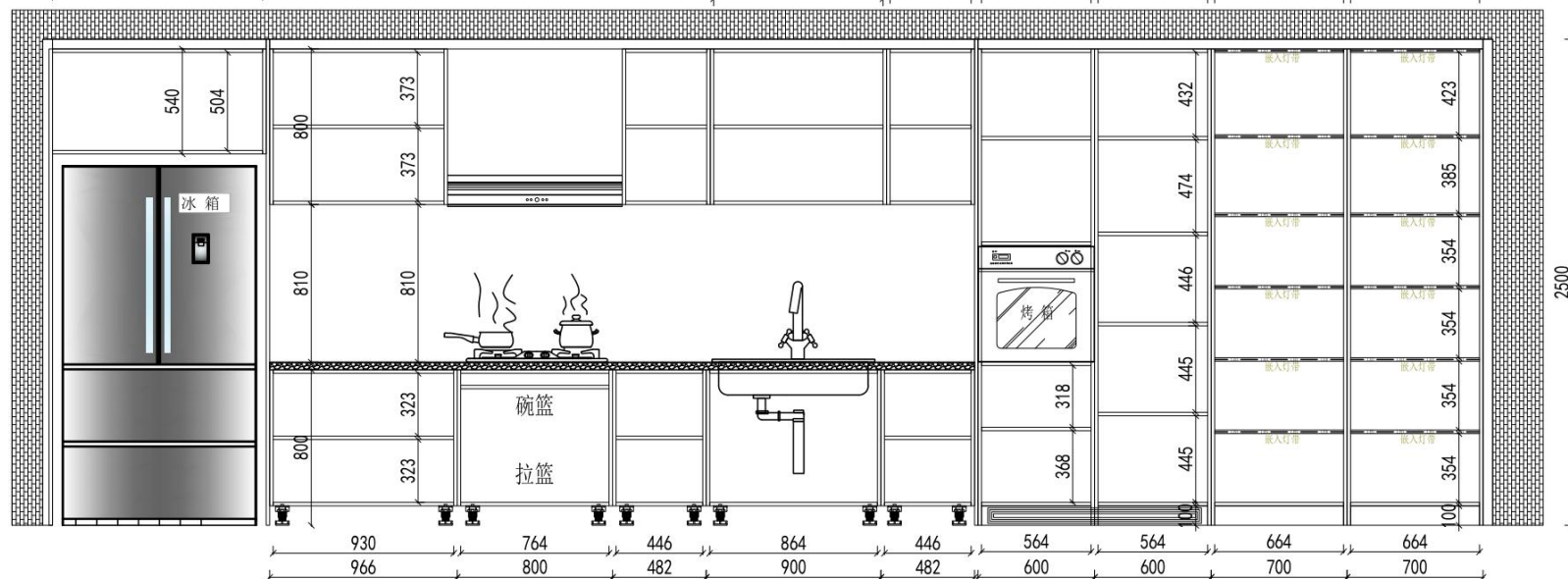
1F厨房结构图
