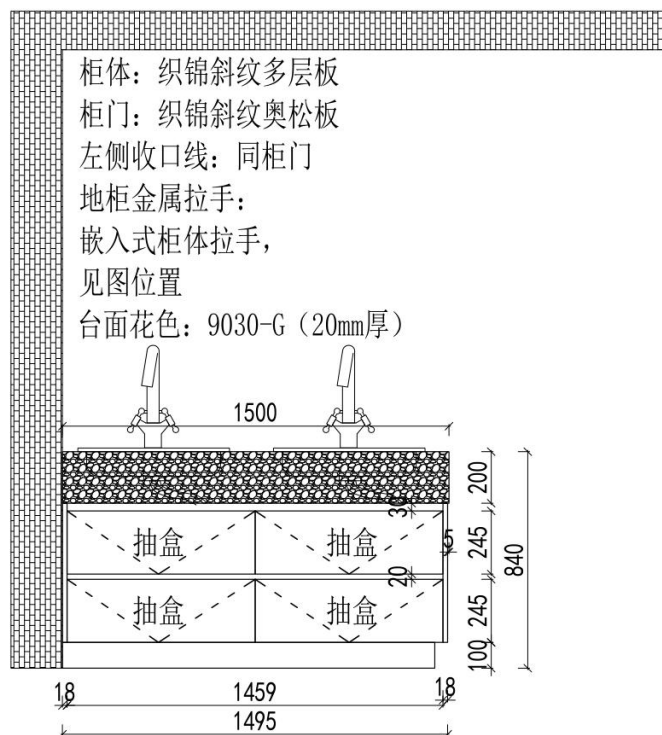
2F卧室3卫生间外视图
