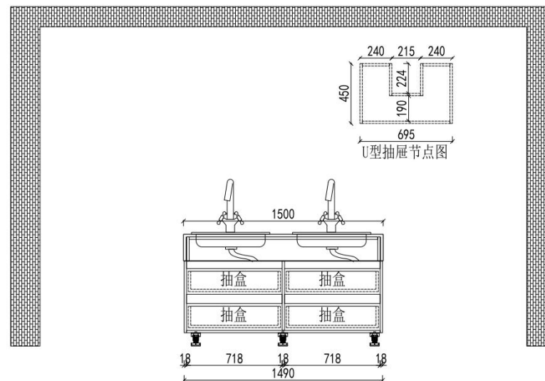
2F主卫结构图
