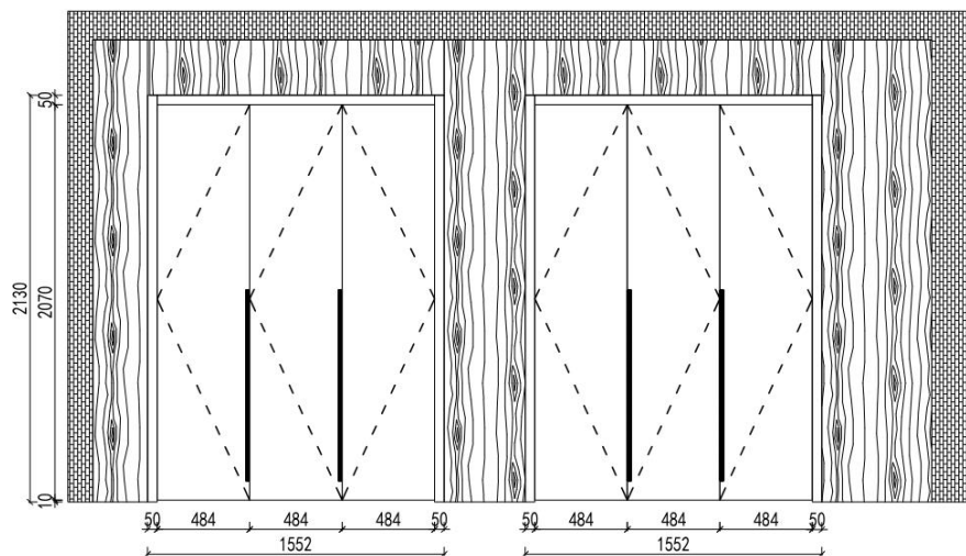
1F客厅衣柜外视图
