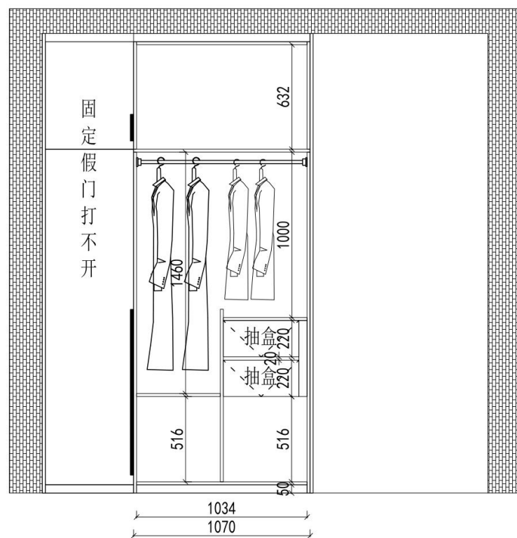
2F儿童房衣柜结构图
