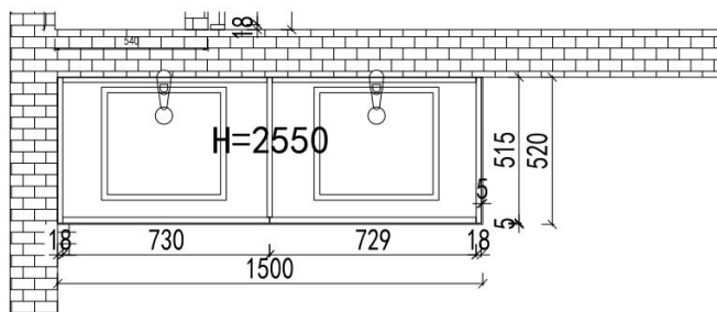
2F卧室3卫生间俯视图
